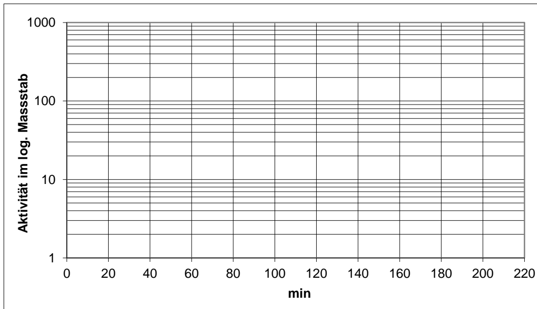
Fig. 1: Uran mit Neutronen bestrahlt. Extraktion mit verdünnter Salzsäure. Zugabe von Bariumchlorid und Fällung mit konz. Salzsäure. Die Halbwertszeiten entsprechen der Steigung (y-Achse als lg einbezogen, also 2 statt 100, da 100 = 10^2 .) Bsp. Die Steigung von RaII ist hier -0.022 (2.2 pro 100 min). Die Halbwertszeit ist gleich \log(e) \cdot \ln(2) / 0.022 = \text{ca. } 14 \text{ min} . Die ungefähre Halbwertszeit zu Beginn der Kurve der Gesamtaktivität wird so abgeschätzt, ebenso die Steigung am Ende der Gesamtaktivität. Wartet man nach der Bestrahlung etwa 1 h, hat man praktisch nur noch die Aktivität der zweiten Substanz. Jetzt kann deren Halbwertszeit schon genauer bestimmt werden. Durch Differenzbildung erhält man auch eine genauere Halbwertszeit der ersten Substanz usw. Wartet man mehr als eine Stunde wird auch praktisch kein AcII mehr nachgebildet aus RaII. Eine Umkristallisation liefert jetzt reines RaIII.
