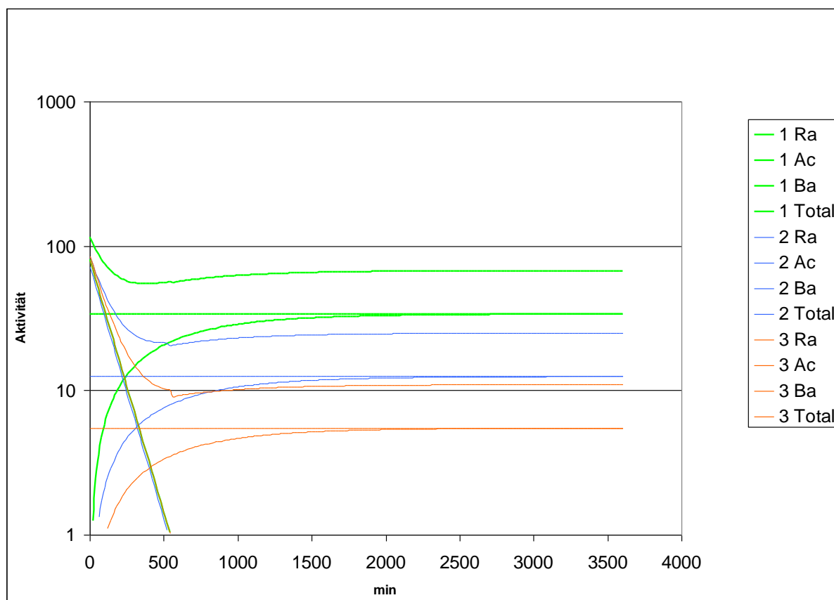
Fig. 2: Der Indikatorversuch mit Zugabe von Ra-228, dessen Aktivität wegen der langen Halbwertszeit während der Messdauer konstant bleibt. Allerdings wird daraus Ac-228 (Kurvenanstieg) nachgebildet. Sein Anteil an der Gesamtaktivität ist im Gleichgewicht ab etwa 2500 min die Hälfte der Gesamtaktivität und wird von dieser abgezogen. Die andere Hälfte ist das konstant strahlende Ra-228 und wird auch von der Gesamtaktivität abgezogen. Es bleiben die reinen Bariumanteile.
